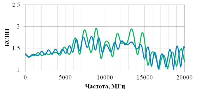
— Порт1 — Порт2
