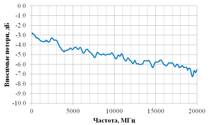
Вносимые потери
