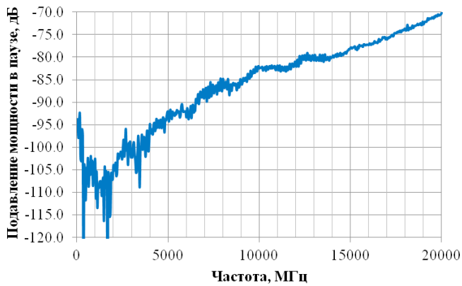
Подавление мощи в паузе
