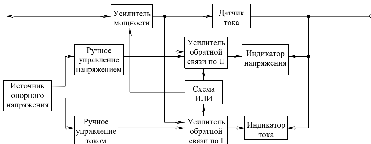
Рисунок 1 – Структурная схема источника питания
