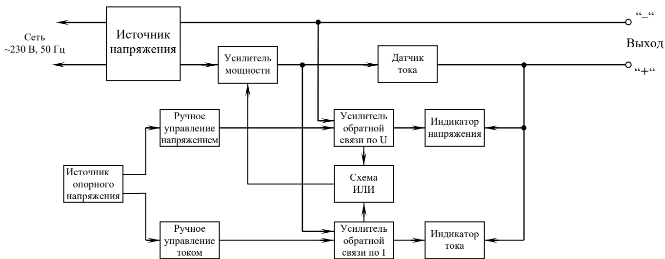
Рисунок 1 – Структурная схема источника питания
